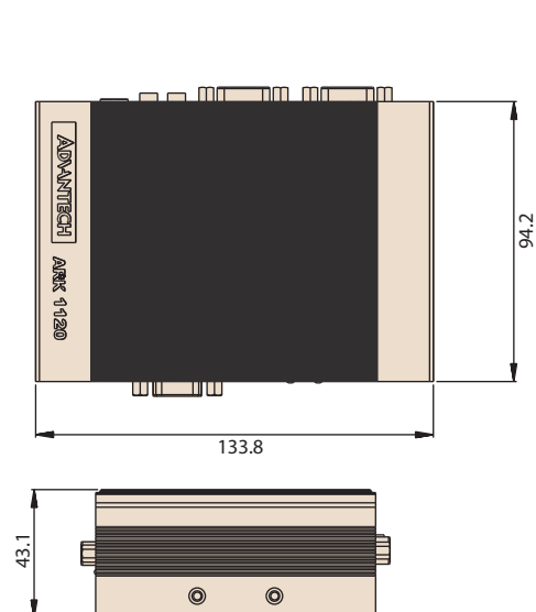
DIN Rail
